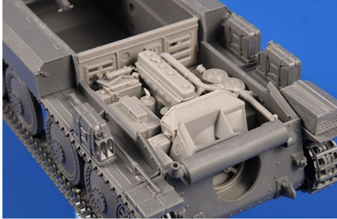
1/35 35CM3142 38(t) 軽戦車E/F型用・エンジンセット・タミヤ
