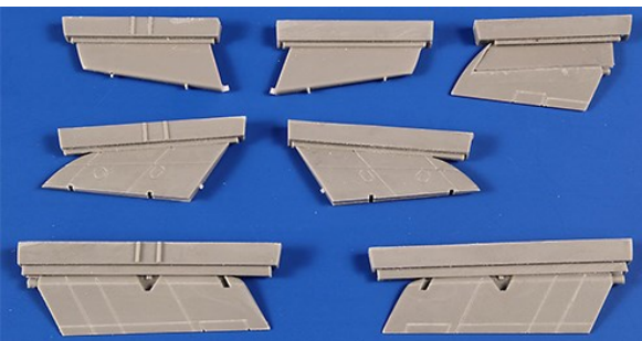
1/72 72CM7440 スーパーマリン スイフト・動翼セット・エアフィクス
