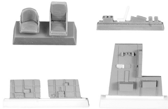
1/72 72CM7425 ロッキード・ハドソンMk.I/V用コクピットセット(エッチング計器板付き)
