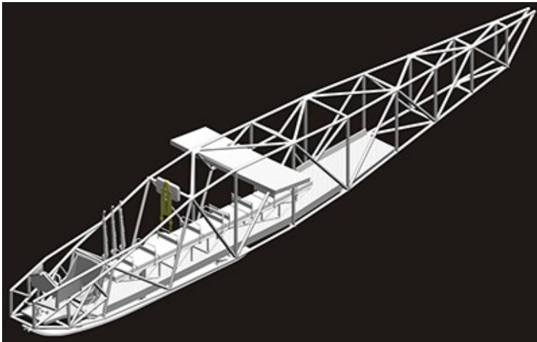
鋼管ハブ張り構想を持つ本機の胴体部はフレームや座席などを細かく再現しています。
