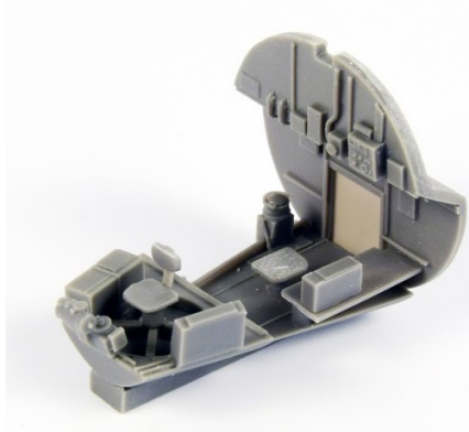
1/72 72CM7384 米・ボーイングB-17G爆撃機・機首爆撃照準席・エアフィクス
